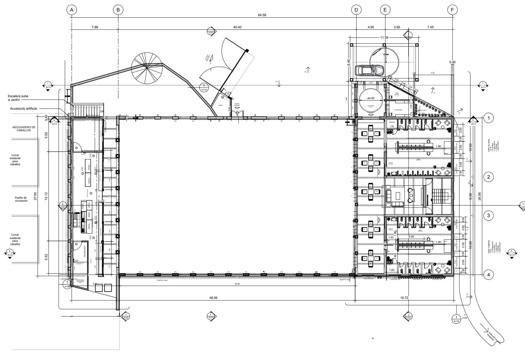
PLANTA ARQUITECTONICA
