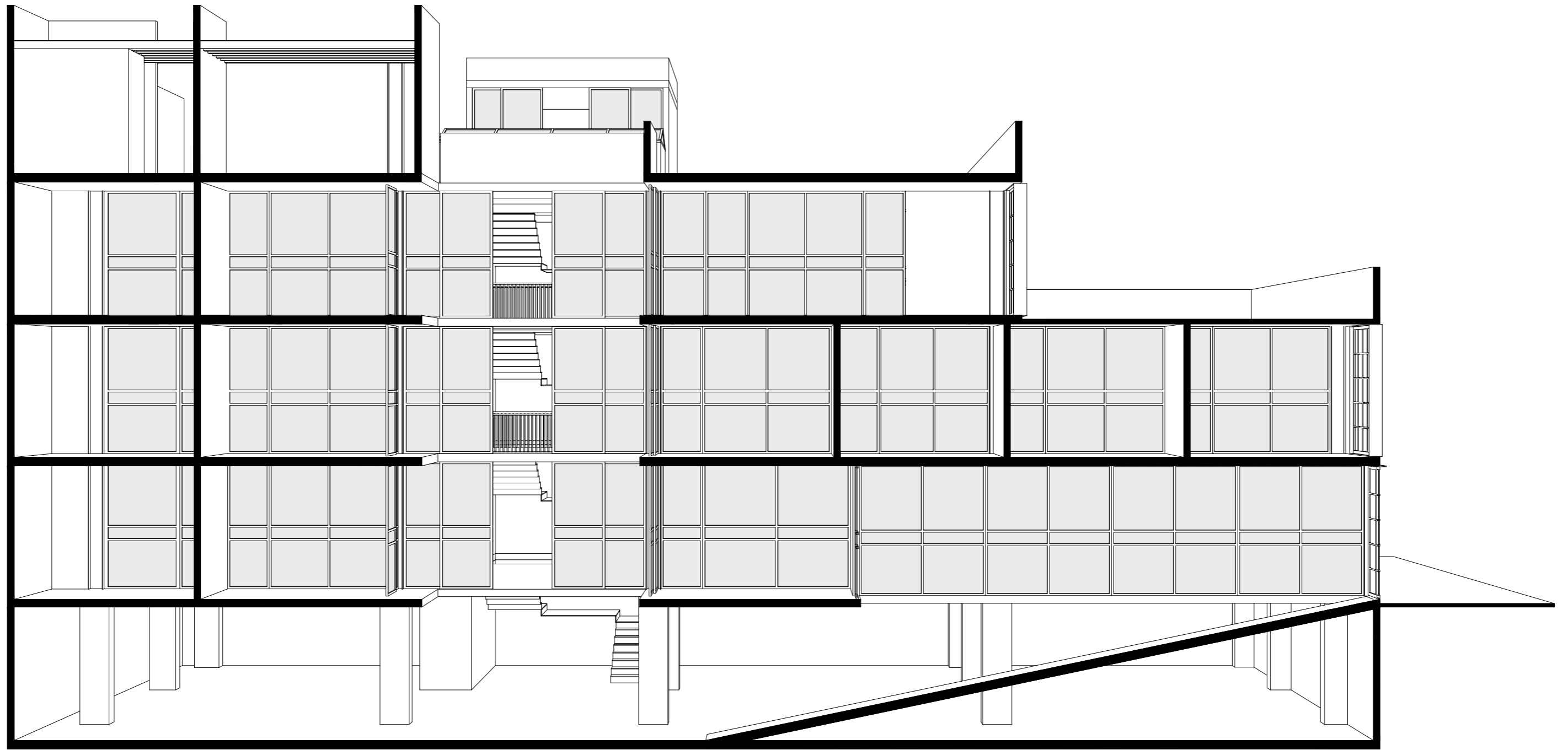
sección esquemática
